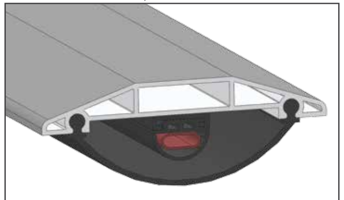
Sicherheitsschließkante 8,2 kOhm
