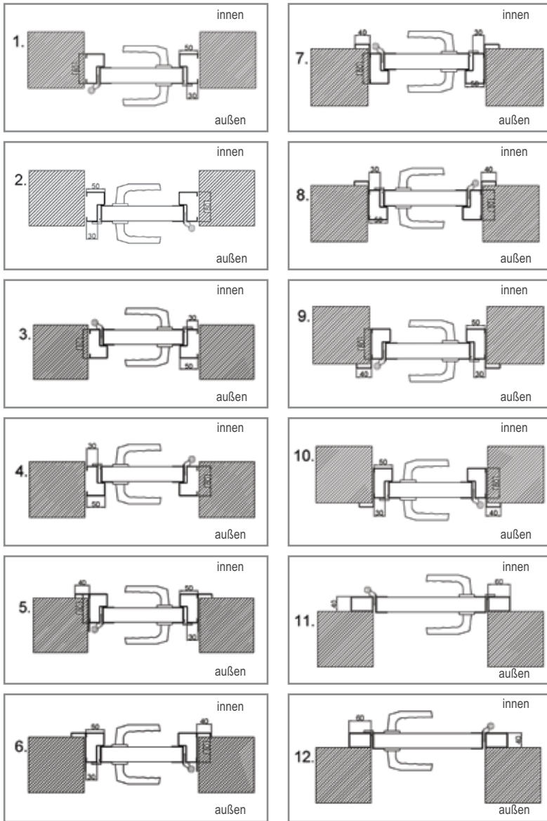
Türzargen
