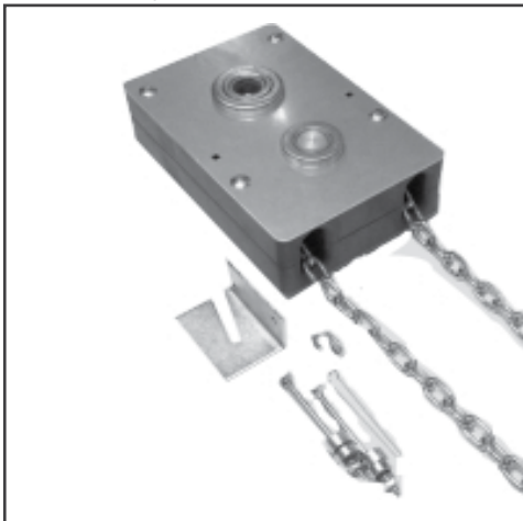
Handkettengertriebe
